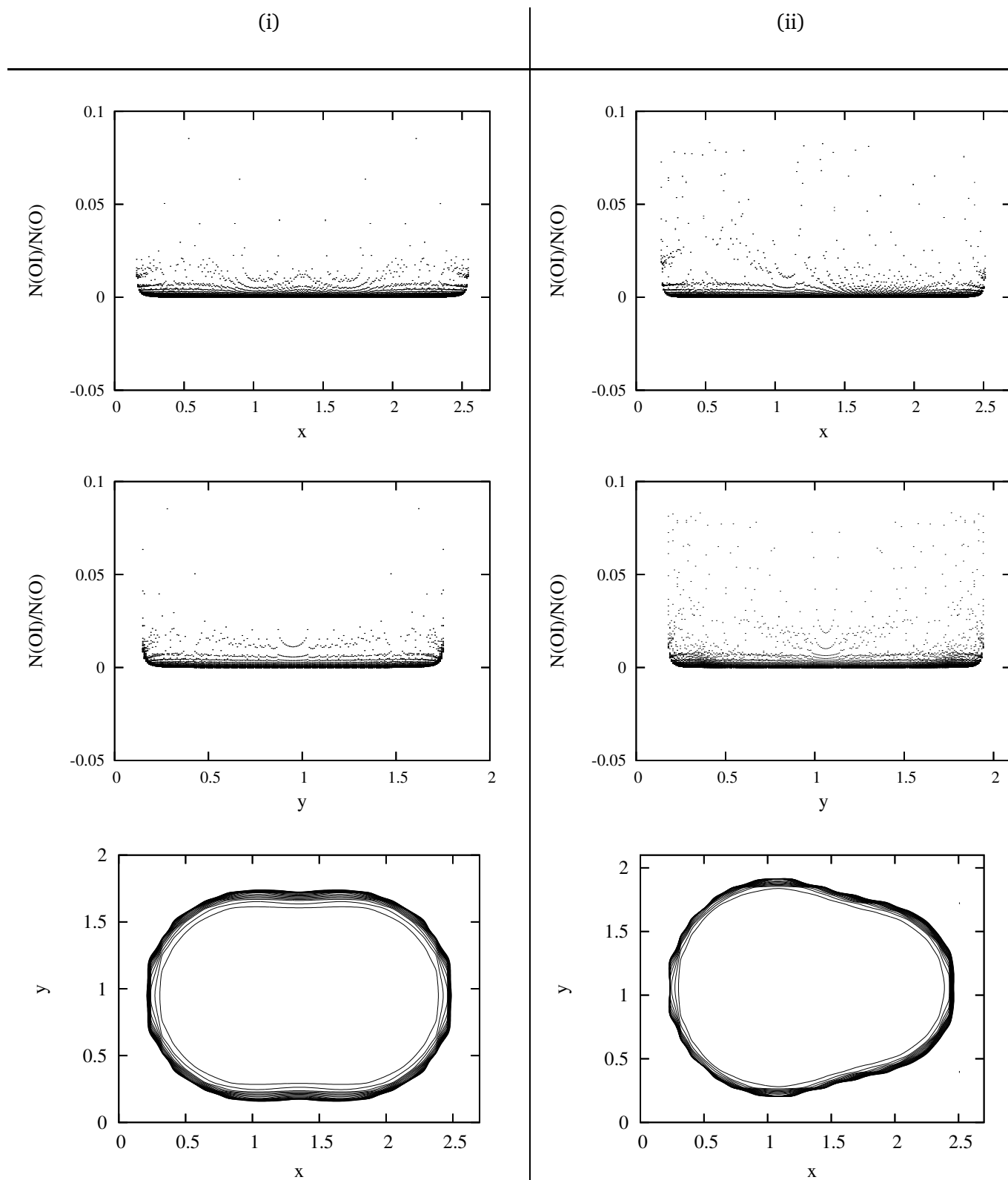
Figura 12. Fracción de ionización del OI para los modelos i y ii (tabla 7). Los ejes x y y están dados en unidades del radio de Strömgen equivalente, R . Se presentan los valores de esta magnitud en las celdas del arreglo y los contornos de nivel en el plano x - y .
